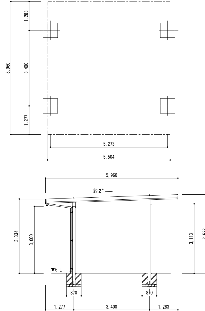
■基礎配置図
