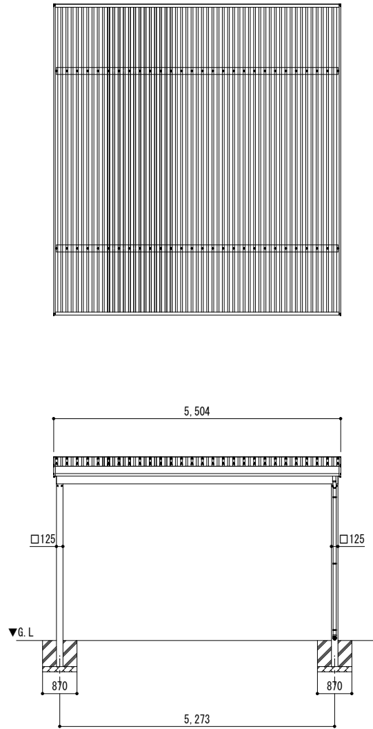
■姿図
